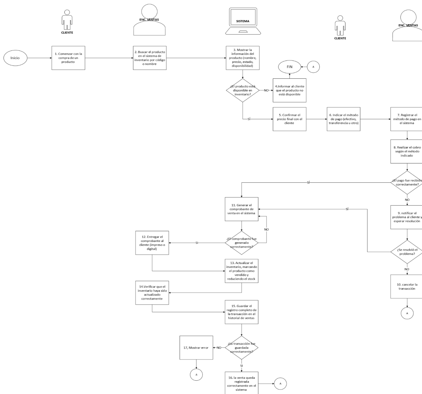
Proceso 2: Proceso de facturación y registro de venta
