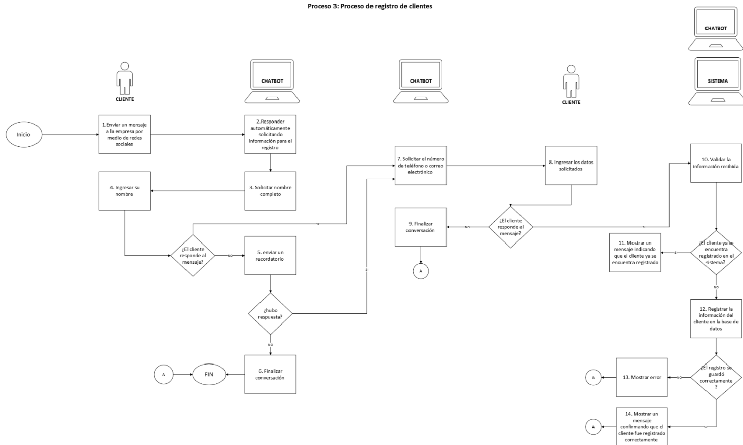
Proceso 3: Proceso de registro de clientes
